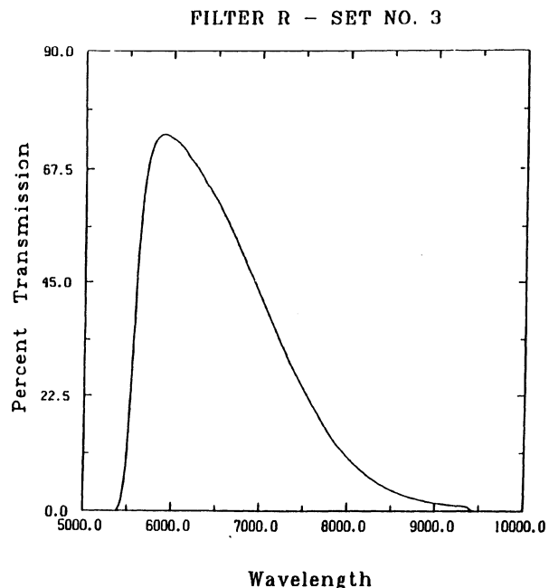
FIG. 49. The transmission characteristics of the R filter: 2 mm KG 3+2 mm OG 570.
